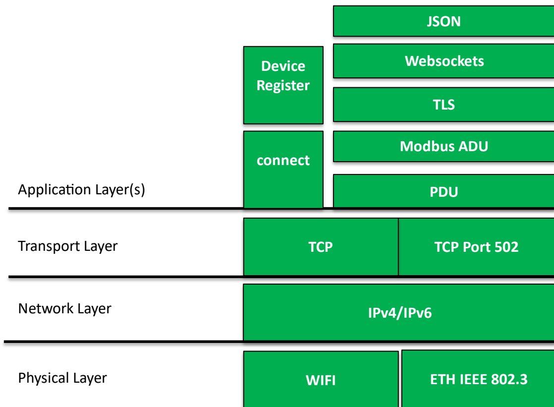
Abbildung 27: Resultierende Protocol Layer aus der Kombination von Modbus TCP und OCPP, eigene Darstellung
