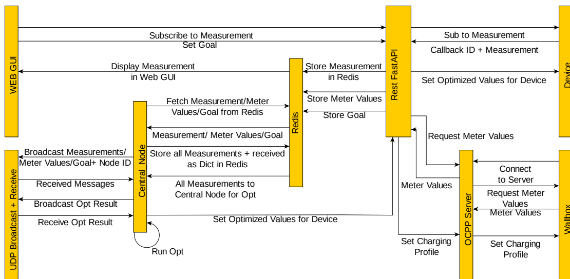
Abbildung 17: Ablaufdiagramm der entwickelten Software, eigene Darstellung
