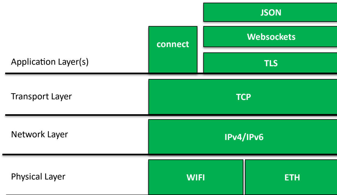
Abbildung 16: Protocol Layers des OCPP, eigene Darstellung nach [32]
