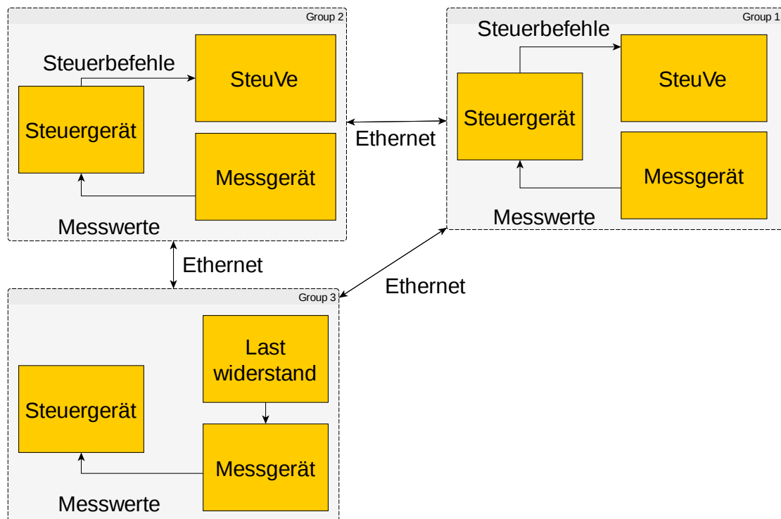
Abbildung 30: Demonstratornetzwerk, eigene Darstellung.
