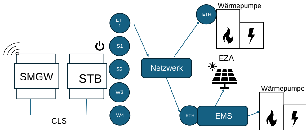
Abbildung 8: Steuerungskonzept 7: 1-4 SteuVE digital plus EMS, eigene Darstellung nach [3].
