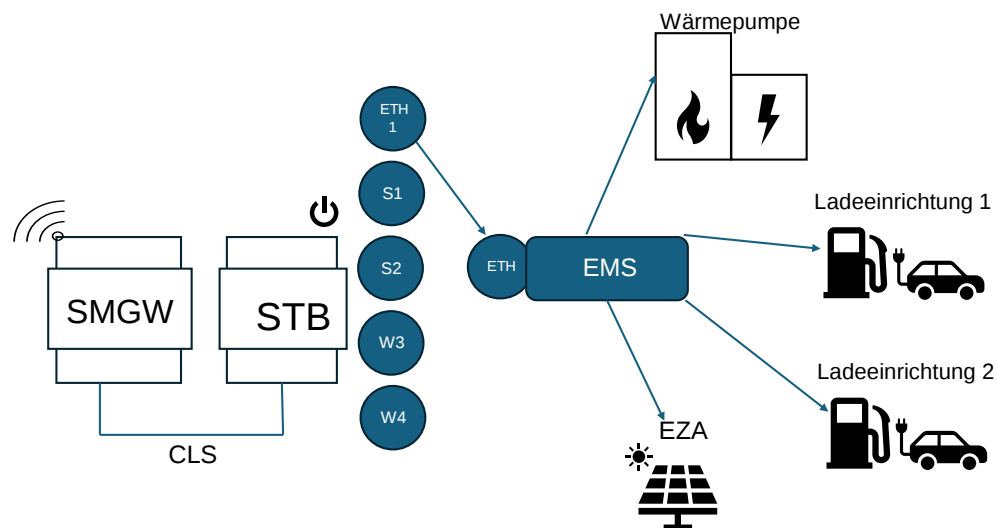
Abbildung 4: Steuerungskonzept 3: EMS Digital, eigene Darstellung nach [3].
