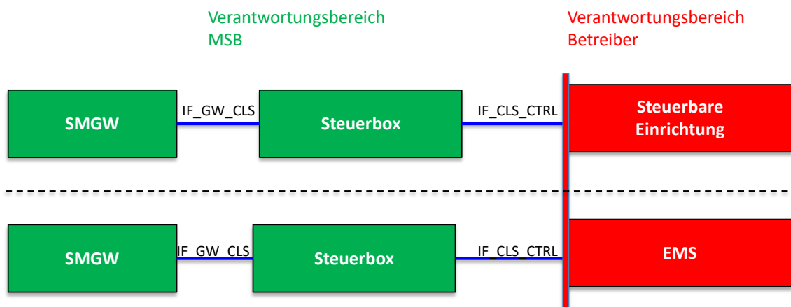
Abbildung 10: Verantwortungsbereiche Messstellenbetreiber und Anlagenbetreiber, eigene Darstellung nach [3].
