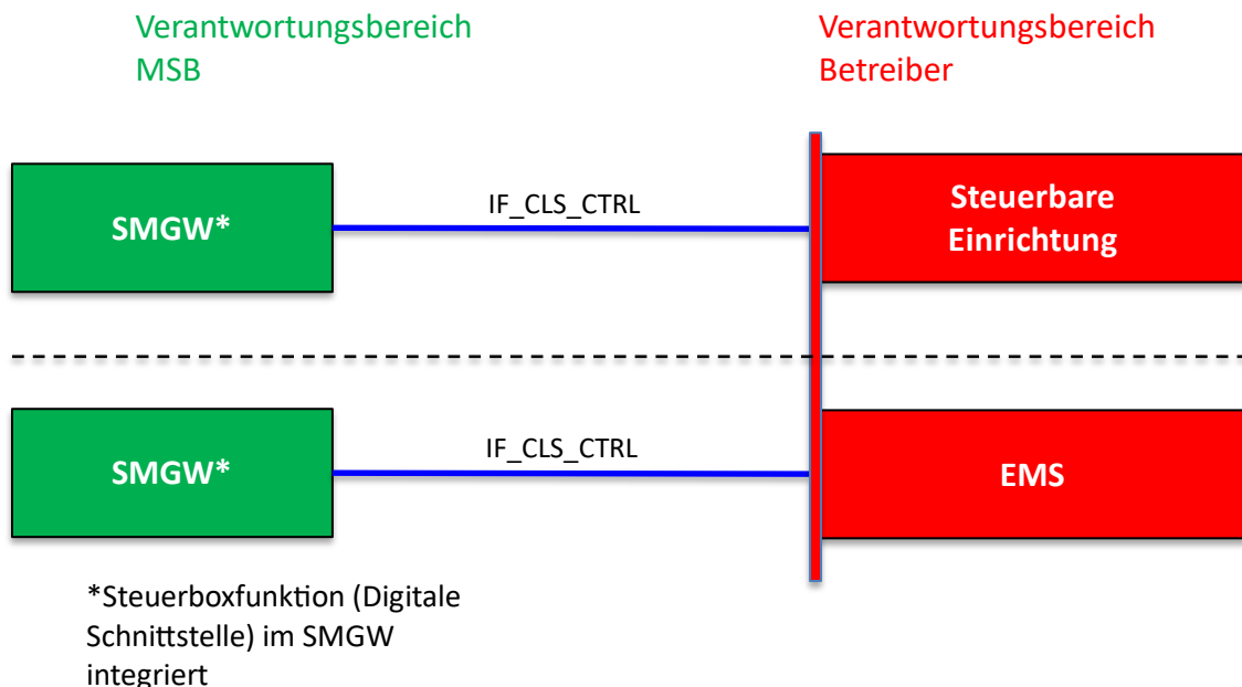
Abbildung 11: Verantwortungsbereich MSB und Betreiber der Anlage bei Integration der Steuerbox in das SMGW, eigene Darstellung nach [3].
