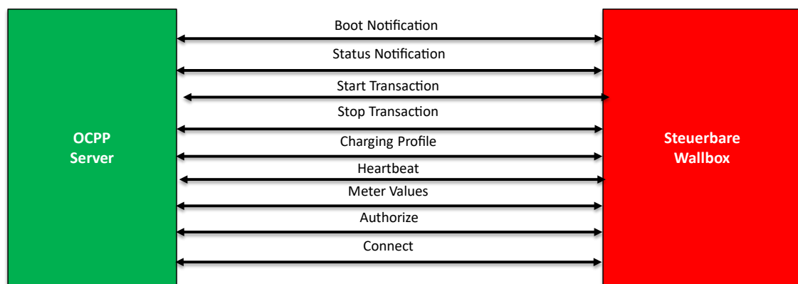
Abbildung 15: Funktionen des OCPP, eigene Darstellung nach [32]
