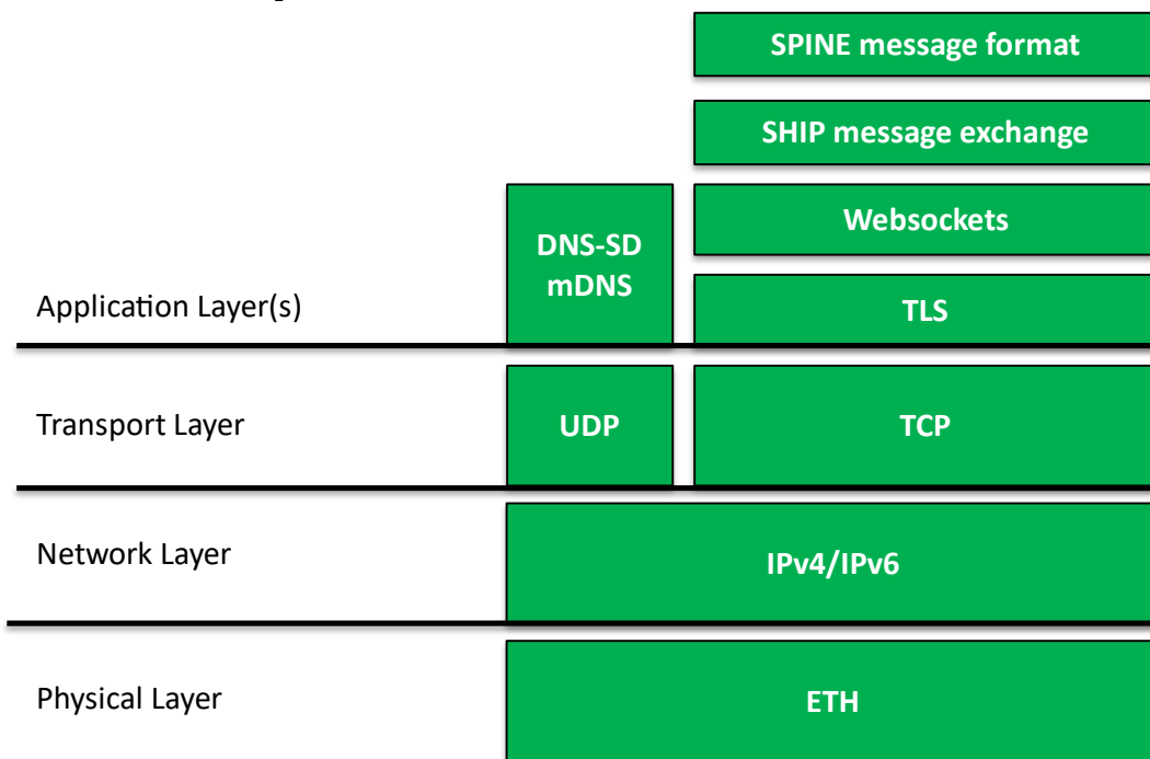
Abbildung 13: Application Layer des EEBUS Protokolls, eigene Darstellung nach [3]
