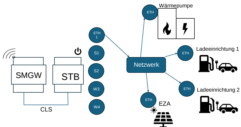
Abbildung 3: Steuerungskonzept 2: 1-4 SteuVE digital, eigene Darstellung nach [3].
