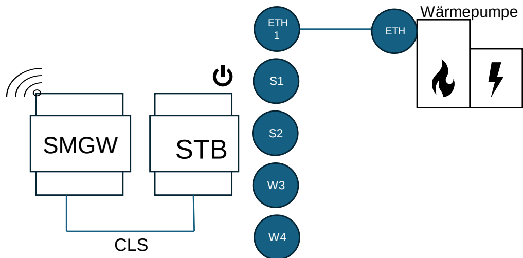
Abbildung 2: Steuerungskonzept 1: 1 SteuVE digital, eigene Darstellung nach [3].
