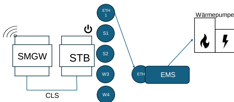
Abbildung 7: Steuerungskonzept 6: EMS digital mit 1 SteuVE, eigene Darstellung nach [3].
