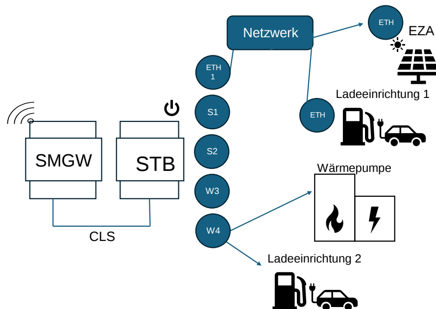
Abbildung 6: Steuerungskonzept 5: 1 EZA digital, 1 SteuVE digital, 1-n SteuVE Relais, eigene Darstellung nach [3].
