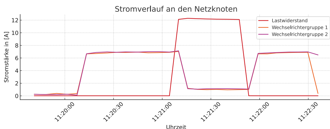
Abbildung 39: Stromverlauf an den Netzknoten in [A], eigene Darstellung
