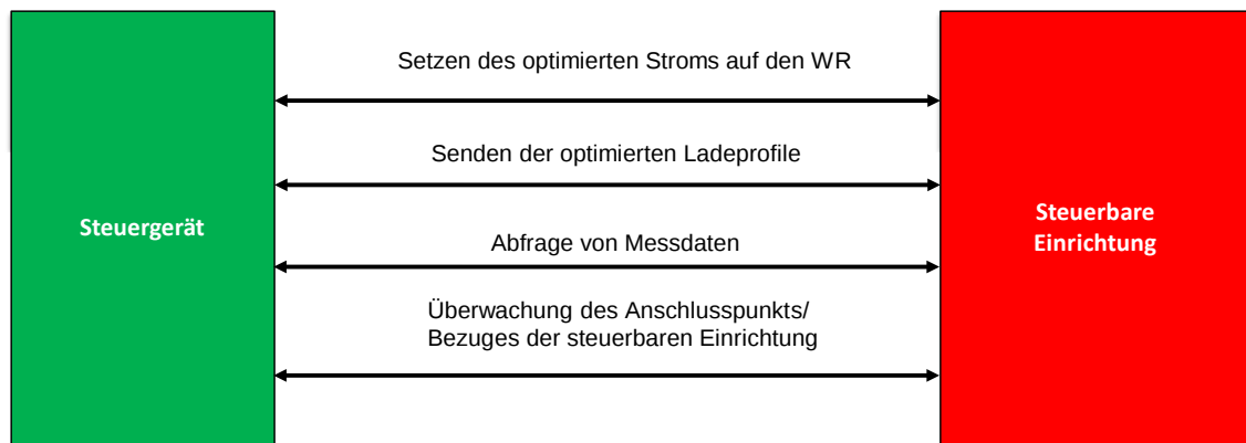
Abbildung 28: Zentrale Funktionen der entwickelten Software, eigene Darstellung.
