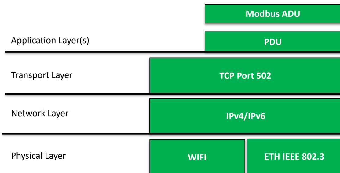
Abbildung 14: Protocol layers von ModbusTCP nach [31]
