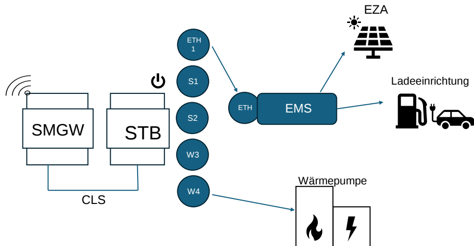
Abbildung 9: Steuerungskonzept 8: 1 digitales EMS plus 1-n SteuVE Relais, eigene Darstellung nach [3].
