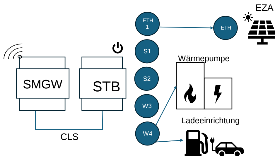
Abbildung 5: Steuerungskonzept 4: 1 EZA digital, 1-n SteuVE Relais, eigene Darstellung nach [3].
