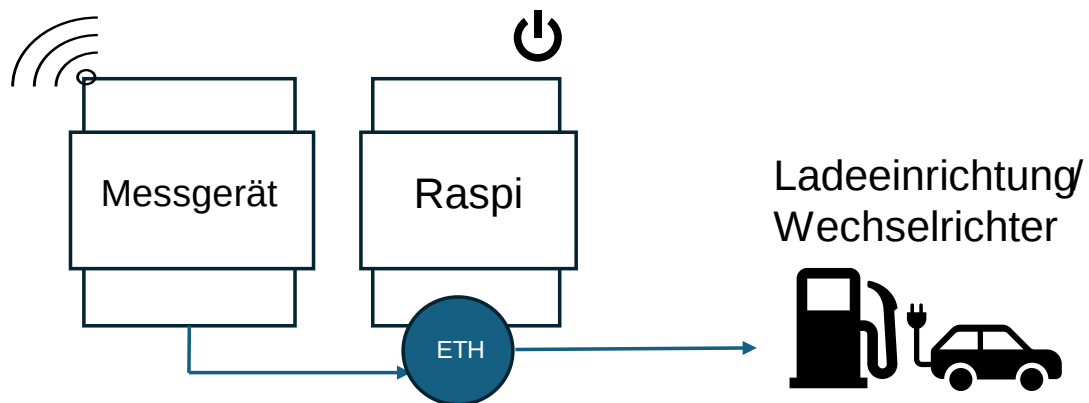
Abbildung 26: Steuerungskonzept Demonstrator, eigene Darstellung
