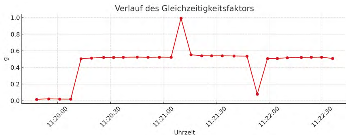
Abbildung 40: Verlauf des Gleichzeitigkeitsfaktors für das Demonstratornetz, eigene Darstellung.
